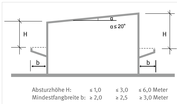
Bild 10: Zulässige Absturzhöhen und erforderliche Fangbreiten bei 0^\circ bis 20^\circ geneigten Flächen
